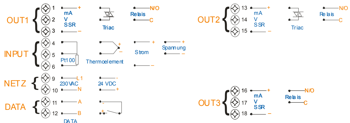
Bild 9 - Rückwärtige Anschlüsse ( 1 / 16 -DIN Geräte)
