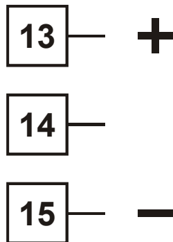
Bild 29 - Options-Steckplatz 2 - Linearspannungs- oder mA DC-Modul
