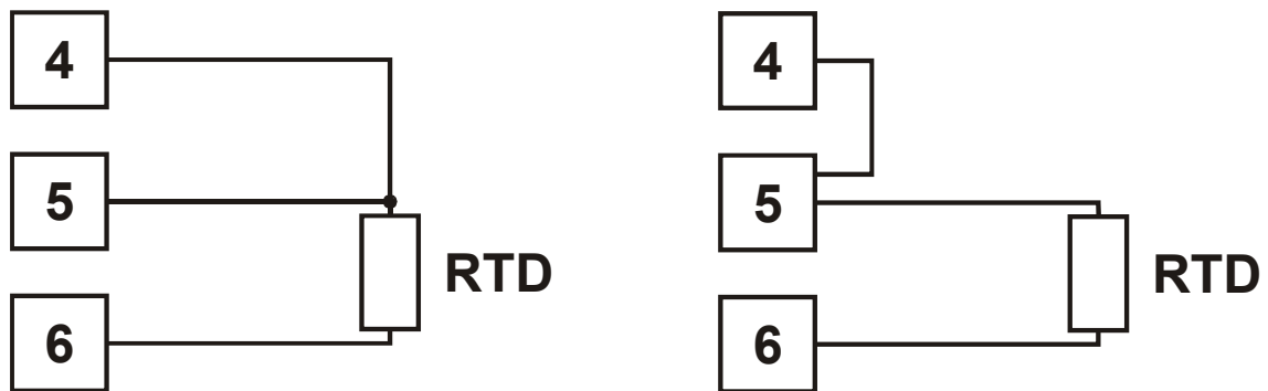
Pt100-Fühler in 3-Leiterschaltung
