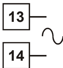
Bild 28 - Options-Steckplatz 2 - Triac-Modul
