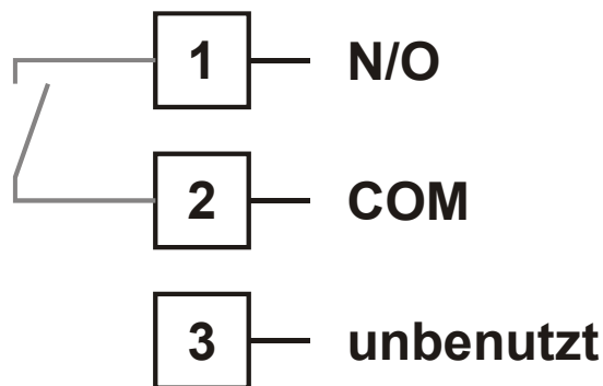
Bild 21 - Options-Steckplatz 1 - Relais-Modul
