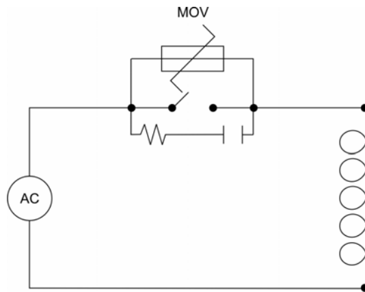
Bild 8 - Störunterdrückung bei Kontakten
