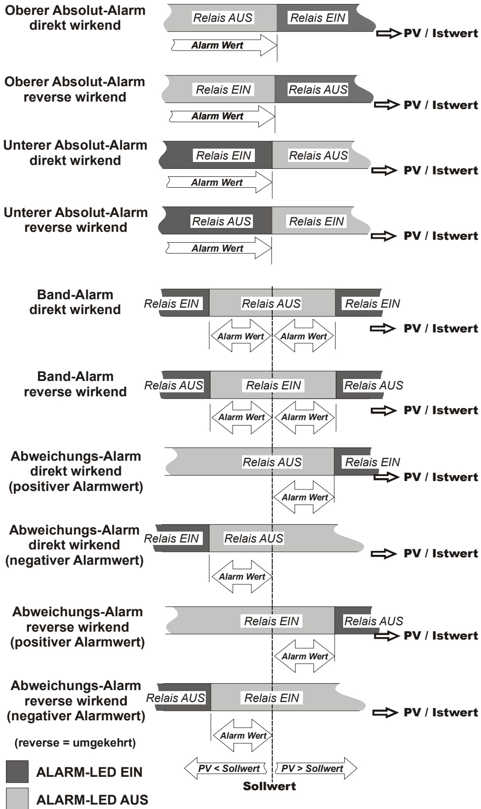
Bild 38 - Alarm-Betrieb
