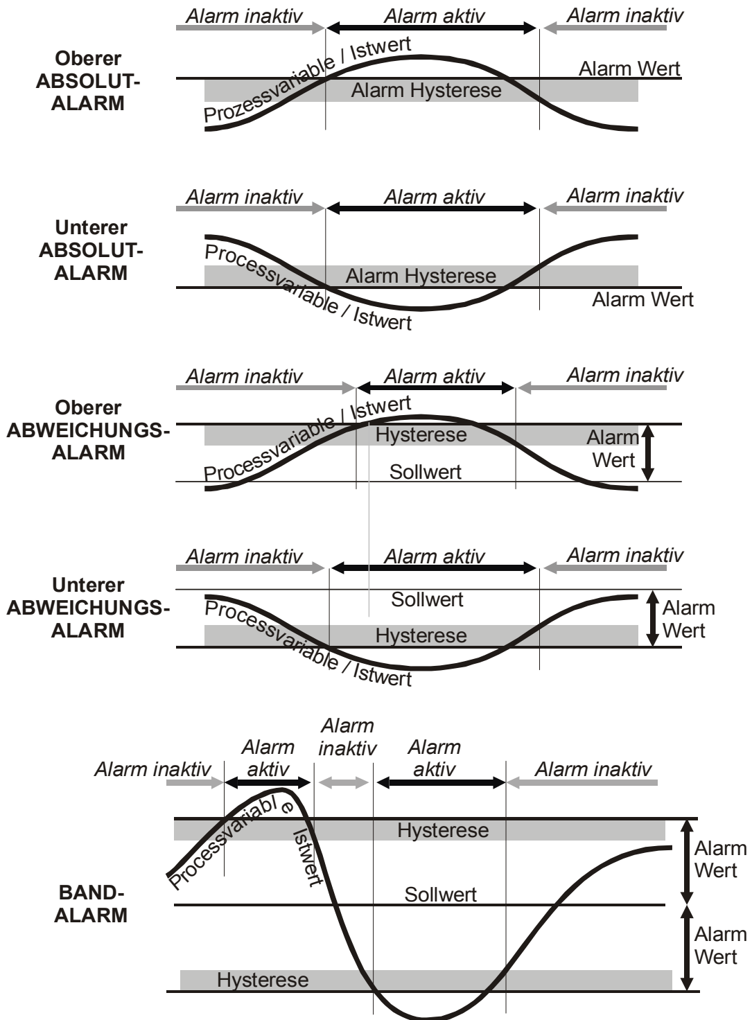
Bild 37 - Alarm-Hysterese-Betriebsart
