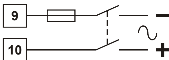
Bild 12 - Anschluss für 24 – 48V AC/DC Versorgung
