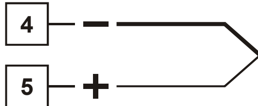
Bild 13 - Anschluss Universal – Eingang: Thermoelement
