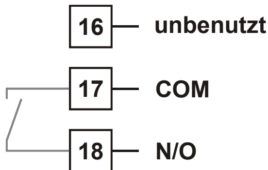
Bild 30 - Options-Steckplatz 3 - Relais-Modul
