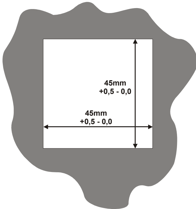
Bild 2 - Montageöffnung
